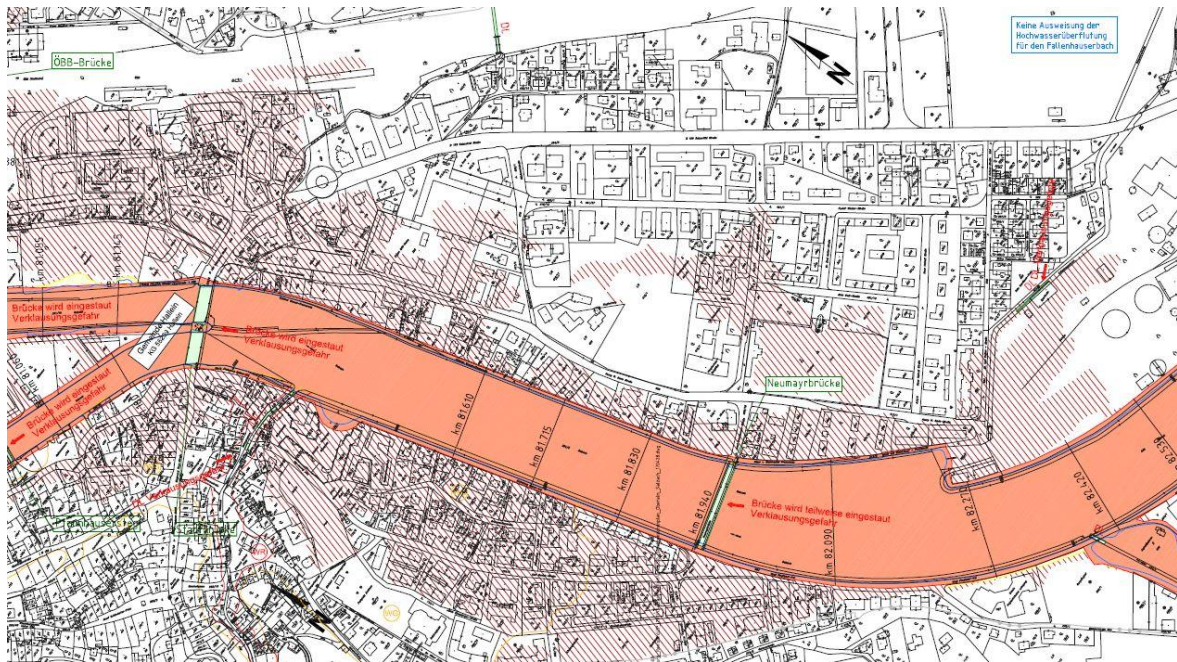
Abbildung 1: Lageplanausschnitt Salzach mit Darstellung der Gefahrenzonen
