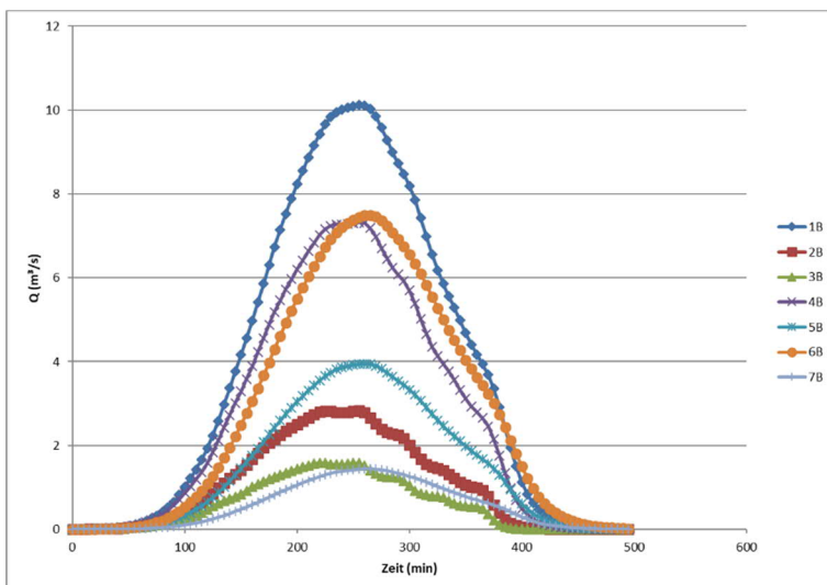
Abbildung 5: Zuflussganglinien HQ300 Mannsbach- Kuchl
