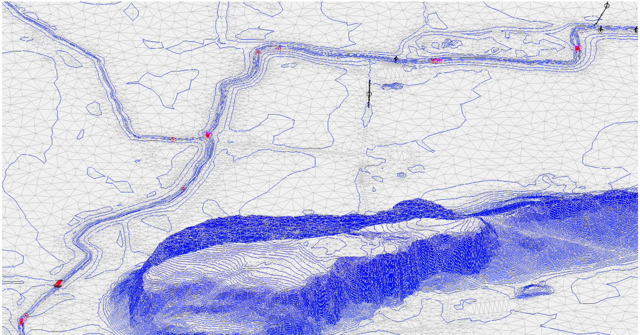
Abbildung 2: Ausschnitt aus Abflussmodell Mannsbach- Kuchl
