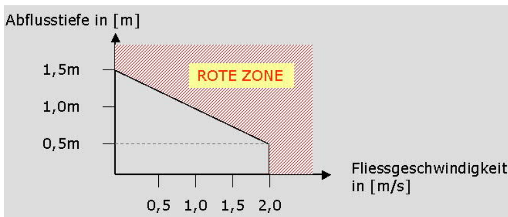
Abbildung 7: Rote Zone nach Wassertiefe und Fließgeschwindigkeit
