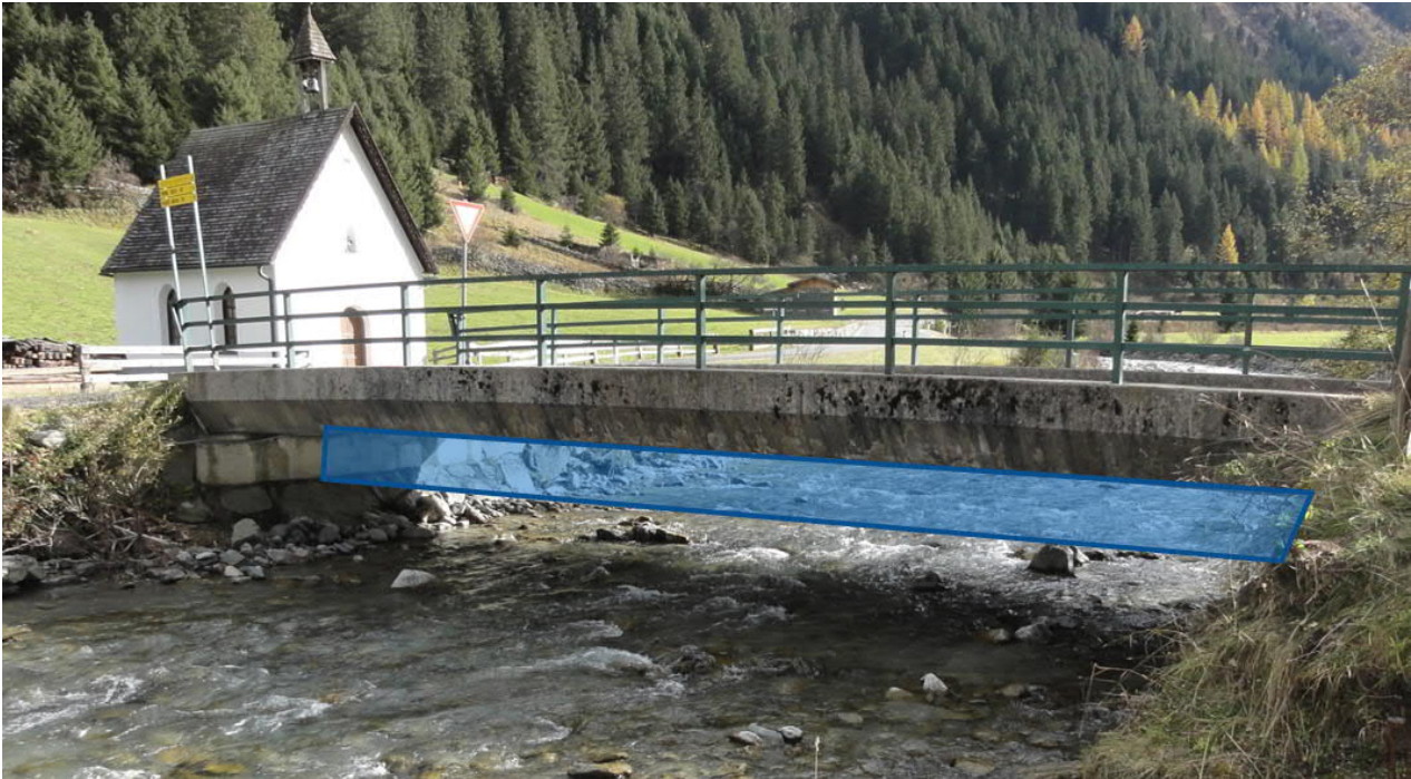
Abbildung 6: Annahme bei Brückenverklausungen. Die Reduktion des Abflussquerschnittes ist in BLAU dargestellt
