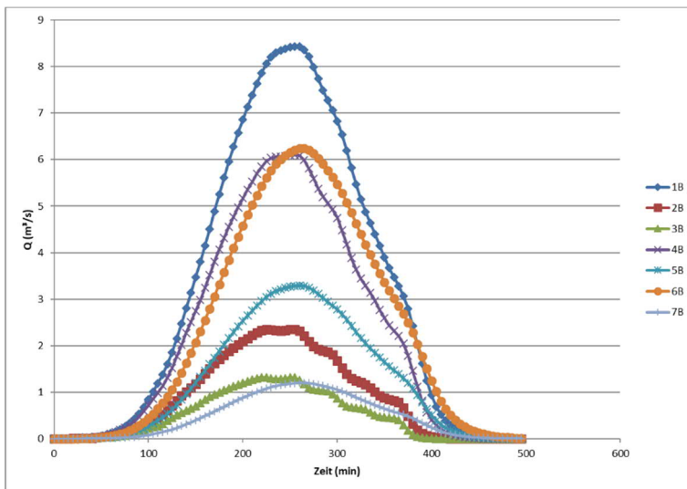
Abbildung 4: Zuflussganglinien HQ100 Mannsbach- Kuchl
