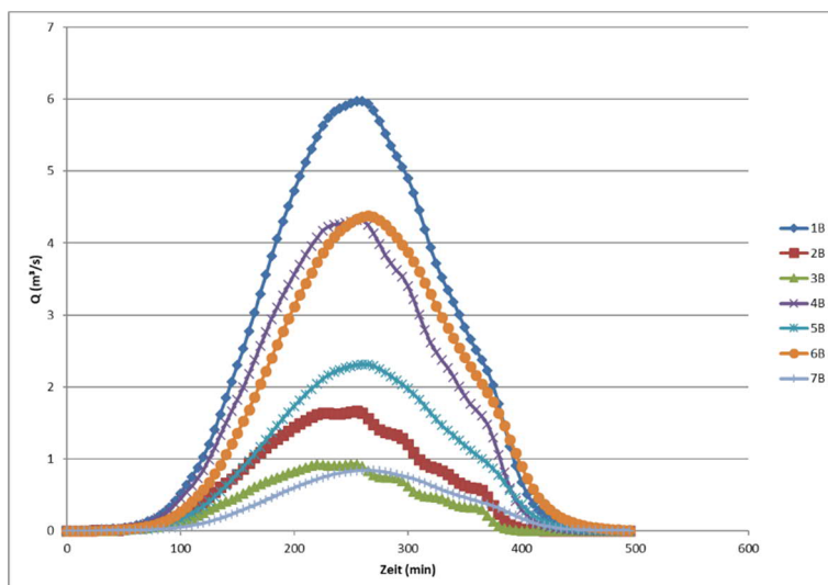
Abbildung 3: Zuflussganglinien HQ30 Mannsbach- Kuchl
