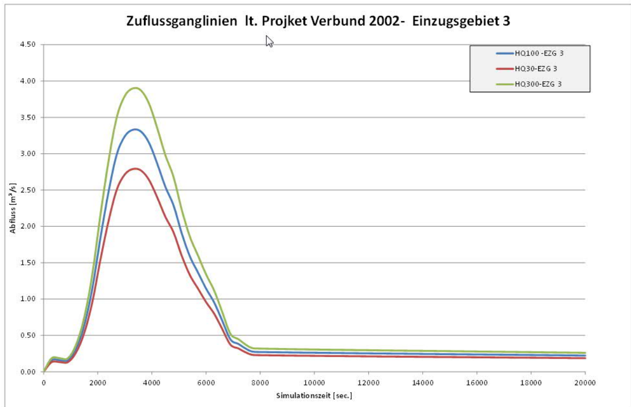
Abbildung 4: Zuflussganglinien Einzugsgebiet3
