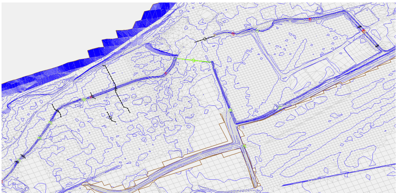
Abbildung 2: Ausschnitt aus Abflussmodell Bruckbergkanal
