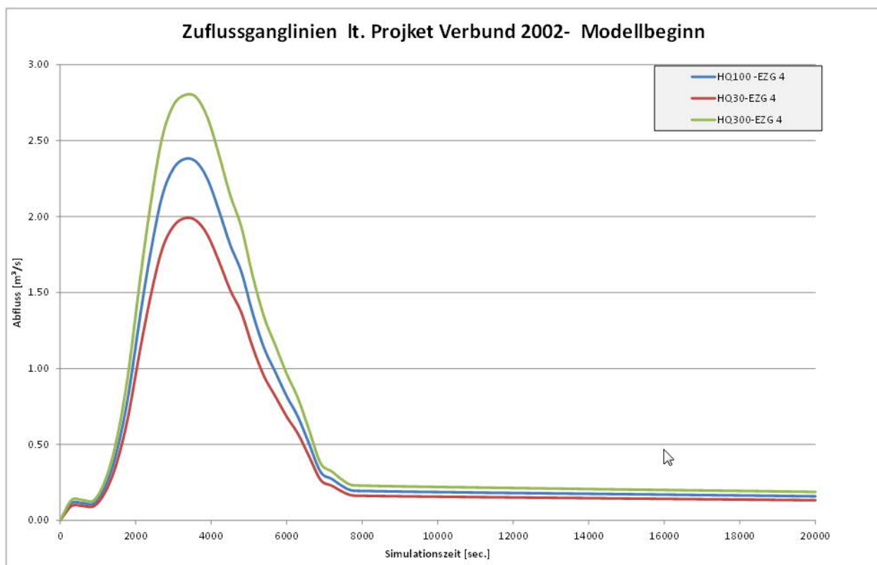
Abbildung 3: Zuflussganglinien Einzugsgebiet 4 – oberes Modellende
