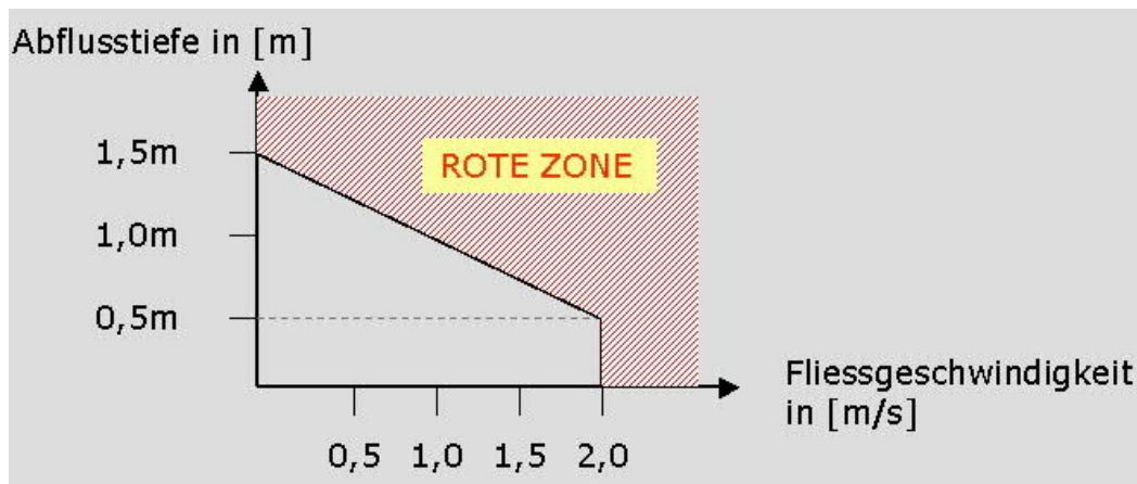
Abbildung 6: Rote Zone nach Wassertiefe und Fließgeschwindigkeit
