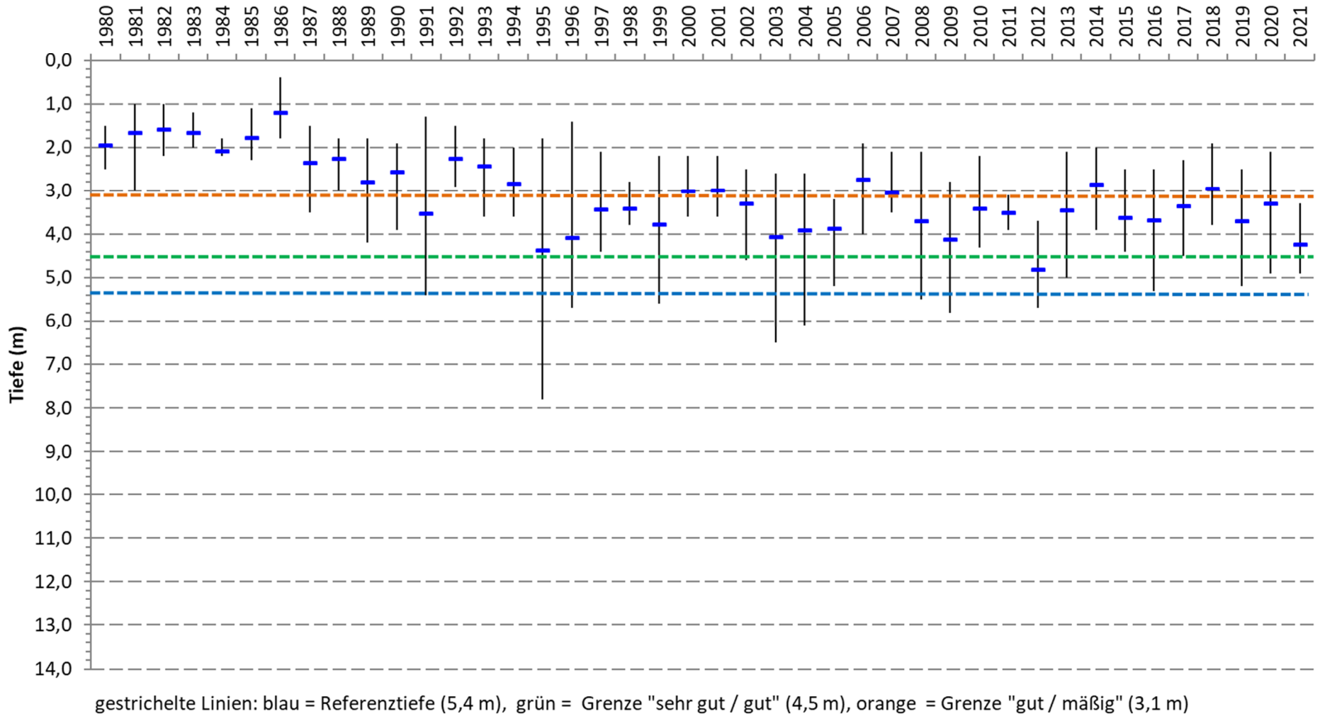
Sichttiefenentwicklung (Jahresmittel, Maximum- und Minimumwerte) ab 1980
