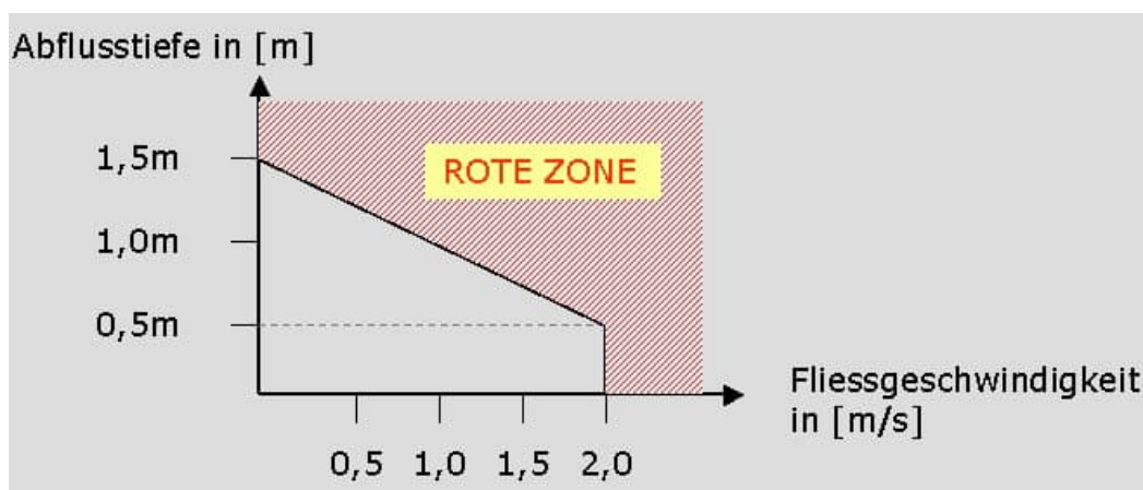
Abbildung 5: Rote Zone nach Wassertiefe und Fließgeschwindigkeit
