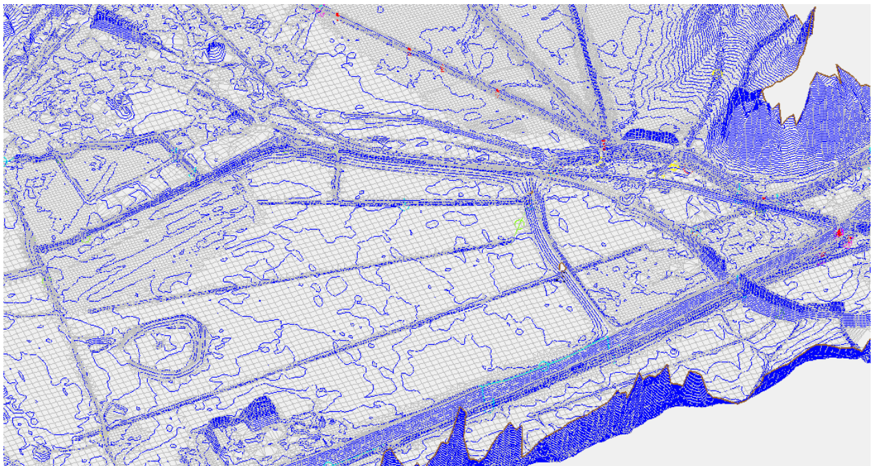
Abbildung 2: Ausschnitte aus Abflussmodell GZP Zeller Becken
