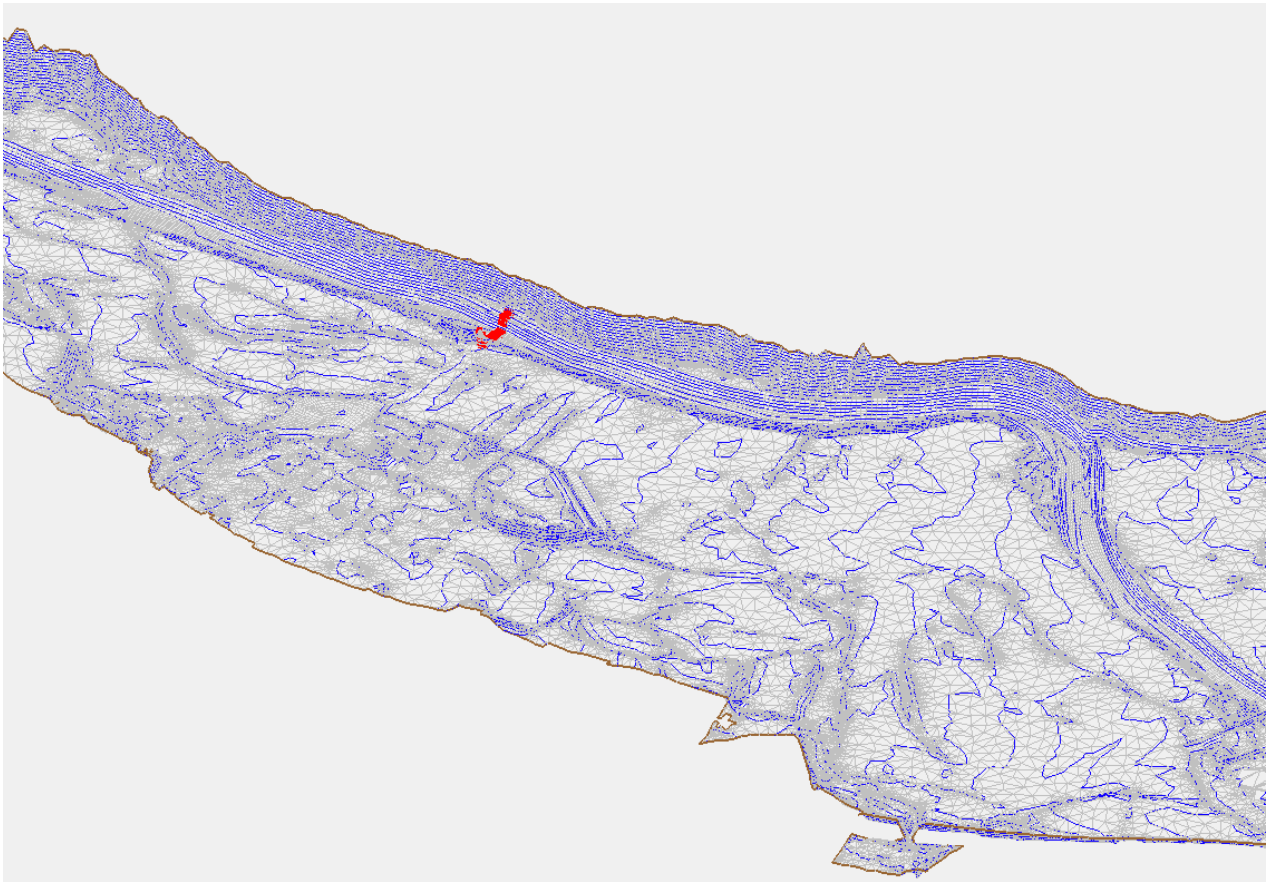
Abbildung 2: Ausschnitt aus dem aktuellen Abflussmodell St. Martin - Saalach
