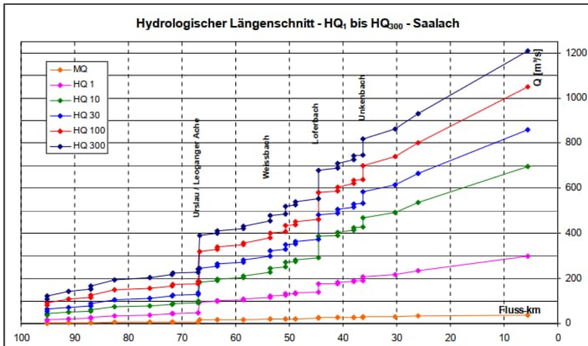
Abbildung 3: hydrologischer Längenschnitt aus GZP Saalach - Pinzgau
