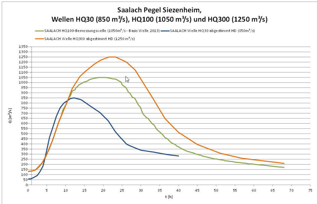
Abbildung 3: Zuflussganglinien Saalach, entnommen aus dem Bericht GZP Wals- Siezenheim 2015-flussbau ic
