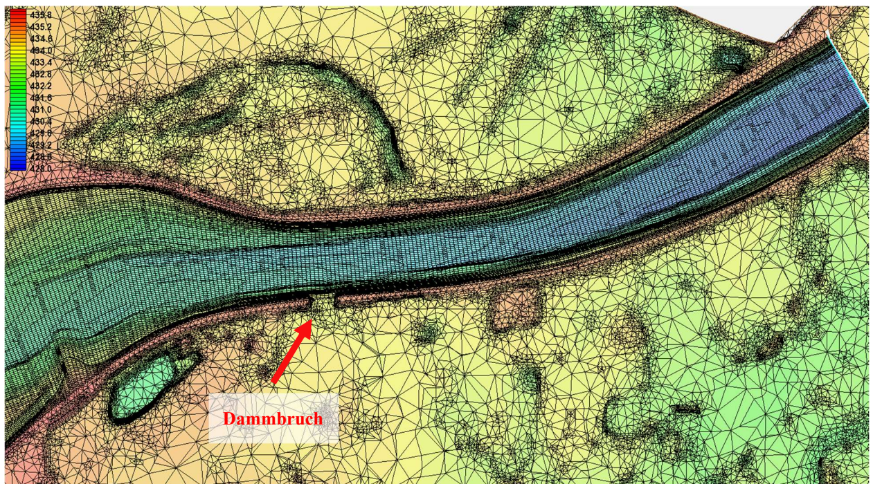
Abb. 14: Dammbruch im Modell
