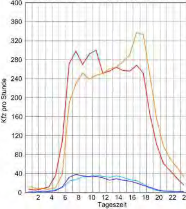
Durchschnittliche Tagesganglinien Mo - Fr
