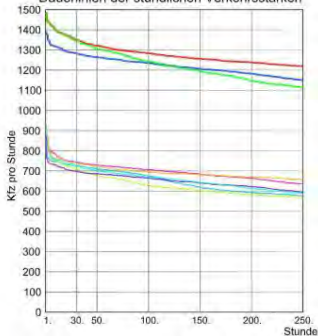
Dauerlinien der stündlichen Verkehrsstärken
