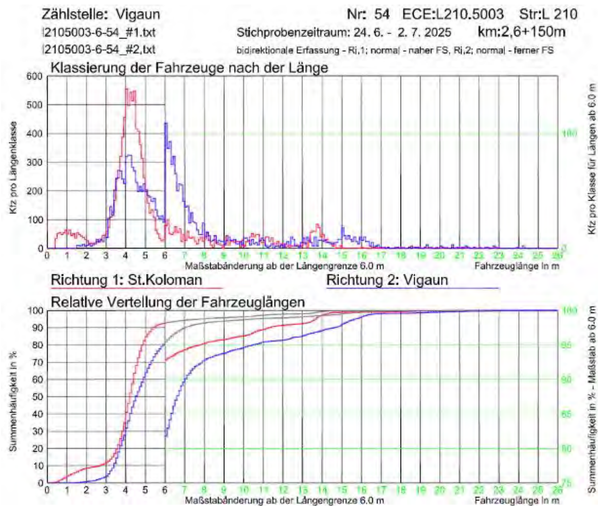
Abbildung 5: Beispiel der Korrektur der Fahrzeuglängen
