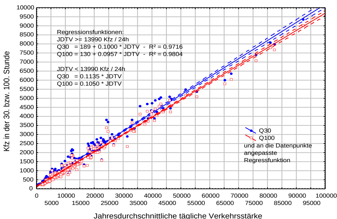
Abbildung 8: Regressionsfunktionen und Grenzen der 90% Konfidenzintervalle des für die Landesstraßen B + L in Salzburg berechneten Zusammenhanges zwischen dem JDTV und der 30. und 100. höchstbelasteten Stunde
