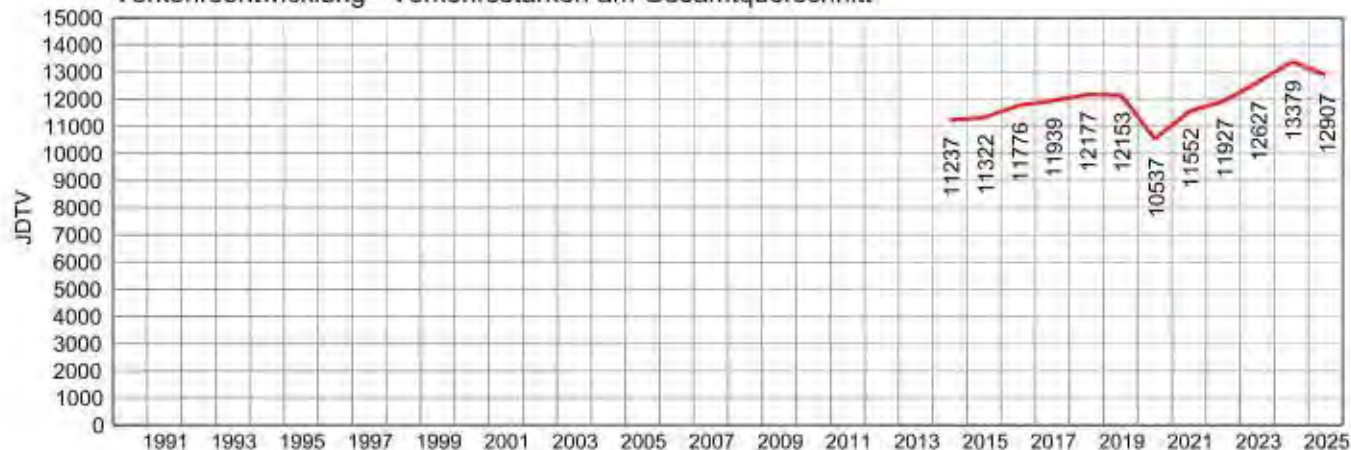
Verkehrsentwicklung - Verkehrsstärken am Gesamtquerschnitt
