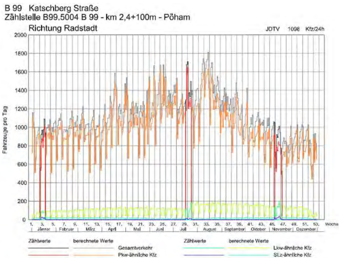
Abbildung 6: Berechnete Jahresganglinie für eine Zählstelle mit drei Stichprobenerhebungen.
