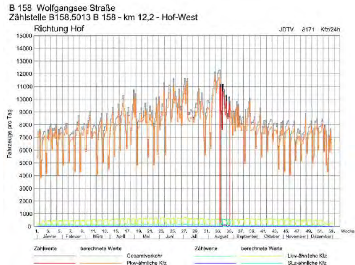
Abbildung 7: Berechnete Jahresganglinie für eine Zählstelle mit einer Stichprobenerhebung
