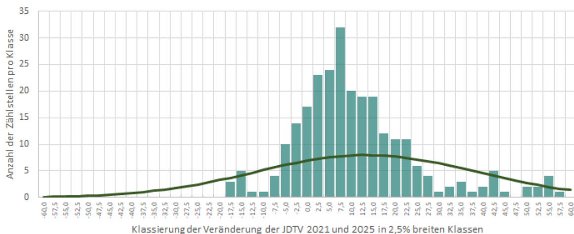
Abbildung 11: Verteilung der relativen Veränderungen der Verkehrsstärken zwischen 2021 und 2025 an allen Zählstellen auf den Landesstraßen B und L und den Autobahnabschnitten in Salzburg und die daran angepasste Normalverteilung
