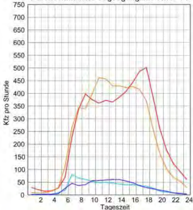
Durchschnittliche Tagesganglinien Mo - Fr
