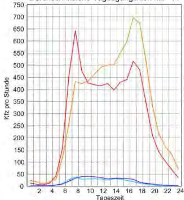
Durchschnittliche Tagesganglinien Mo - Fr
