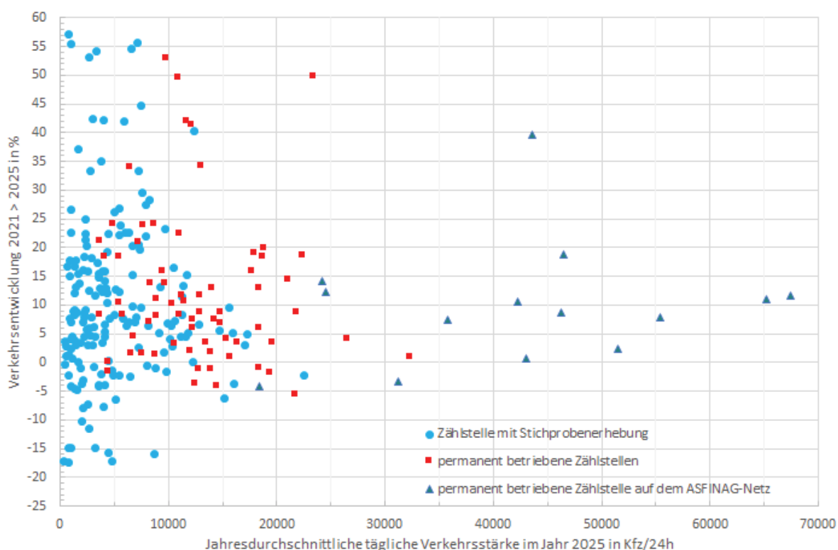
Abbildung 9: Relative Veränderung der Verkehrsstärken im Zeitraum zwischen 2021 und 2025 über dem JDTV mit einer Unterscheidung der Zählstellen nach Erhebungsarten.
