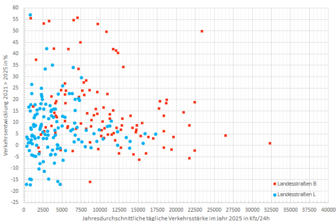
Abbildung 10: Relative Veränderung der Verkehrsstärken im Zeitraum zwischen 2021 und 2025 über dem JDTV mit einer Unterscheidung der Werte nach Landesstraßen B und Landesstraßen L (Die Werte für die Autobahnabschnitte sind in der Abbildung 9 dargestellt).
