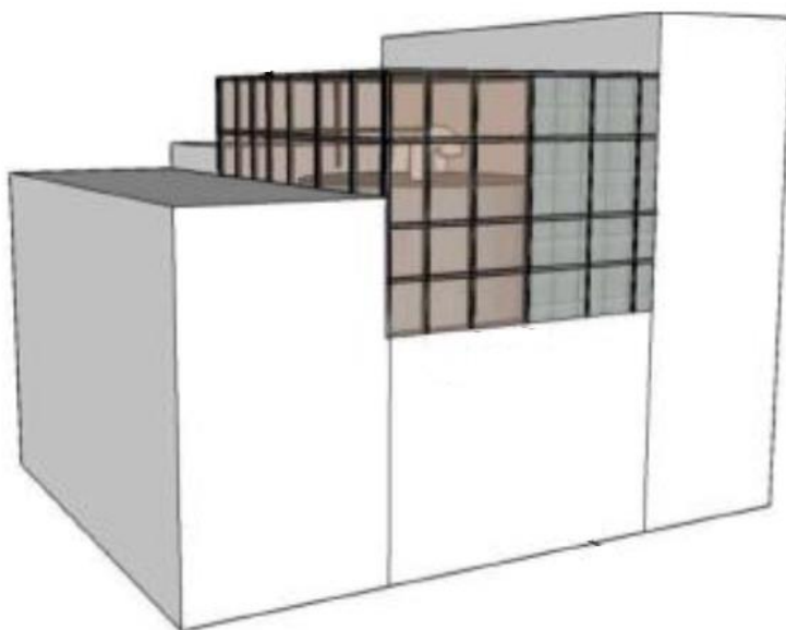
Figure 17. Protection contre la tornade « Noyau Dur » : photo de l'installation actuelle et illustration de la disposition proposée, de type « grilles renforcées », autour de la bache PTR cylindrique.
