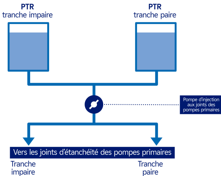
Figure 15. Configuration avant l'installation de la pompe d'injection aux joints « Noyau Dur » (PIJ-ND)
