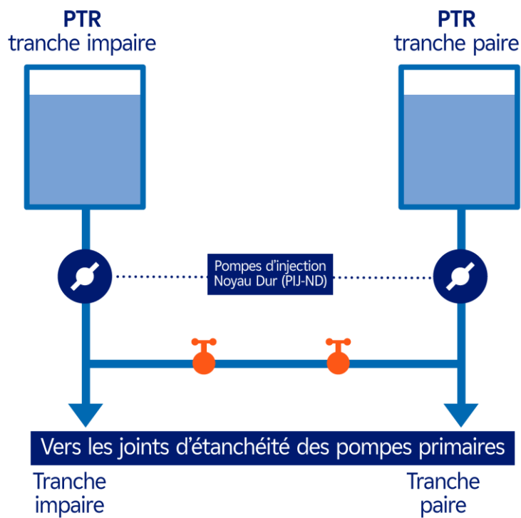
Figure 16. Configuration avec pompes d'injection aux joints « Noyau Dur » (PIJ-ND)
