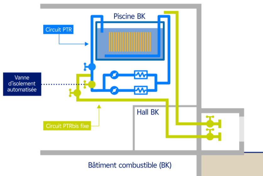
Figure 7. Disposition « Doublement du dispositif d'isolement automatique de la ligne d'aspiration de la piscine BK » : emplacement de la vanne
