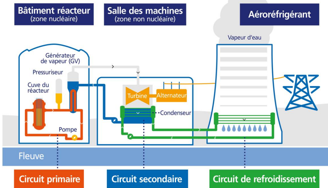
Figure 22. Principes de fonctionnement d'une centrale nucléaire
