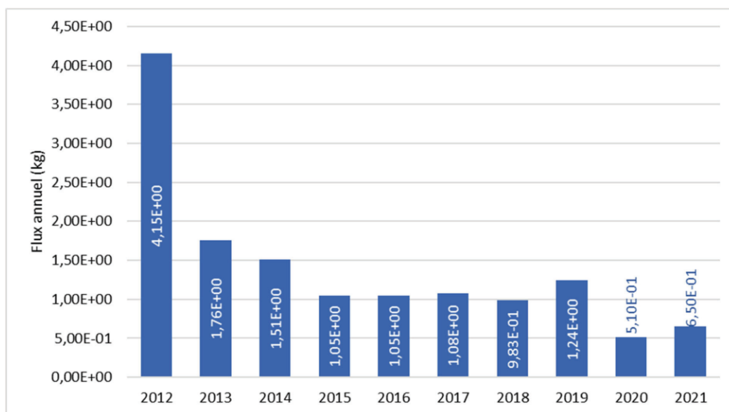
Figure 10 : Rejets annuels d'hydrazine sur la période 2012 – 2021 du CNPE de Saint-Laurent
