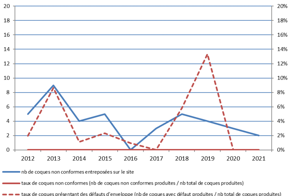
Figure 33: Évolution de la qualité des coques produites sur le CNPE de Saint-Laurent sur la période 2012-2021
