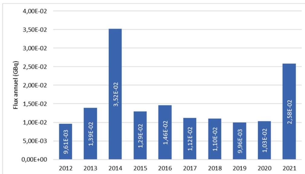
Figure 5 : Activité en iodes rejetée à l'atmosphère par le CNPE de Saint-Laurent sur la période 2012 – 2021 (GBq/an)
