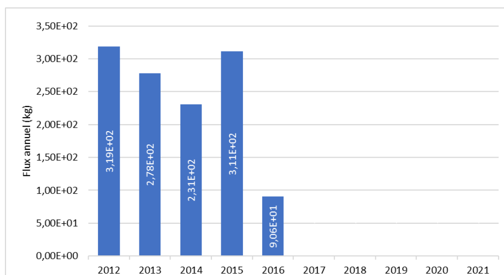
Figure 11 : Rejets annuels de morpholine sur la période 2012 – 2016 du CNPE de Saint-Laurent
