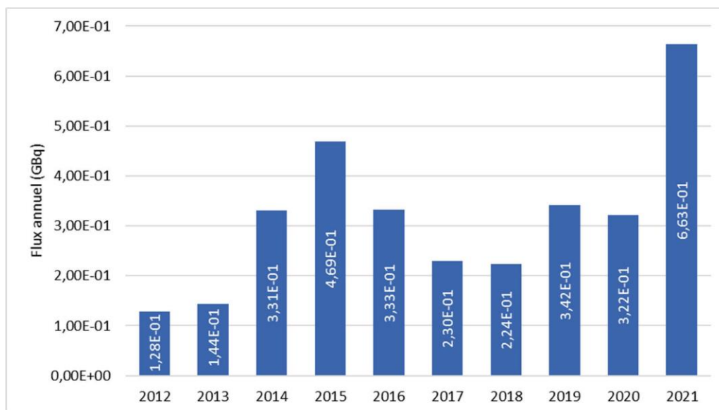
Figure 7 : Activité en autres PF/PA rejetée dans les effluents liquides du CNPE de Saint-Laurent sur la période 2012 2021 (GBq/an)
