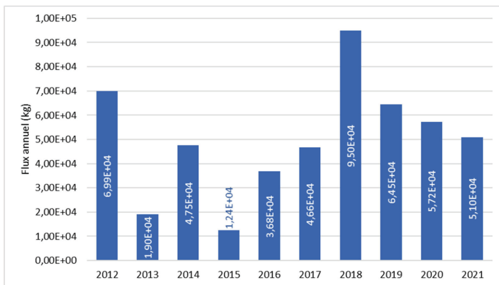
Figure 16 : Rejets annuels des nitrates issus du traitement biocide du CNPE de Saint-Laurent sur la période 2012 – 2021
