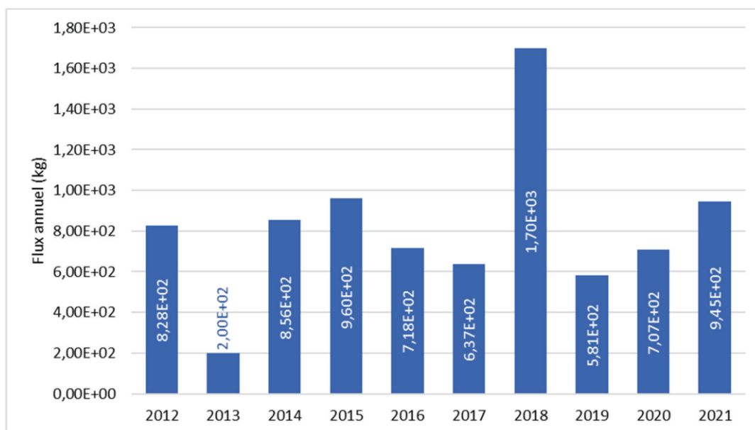
Figure 19 : Rejets annuels de CRT issus des traitements biocides du CNPE de Saint-Laurent sur la période 2012 – 2021
