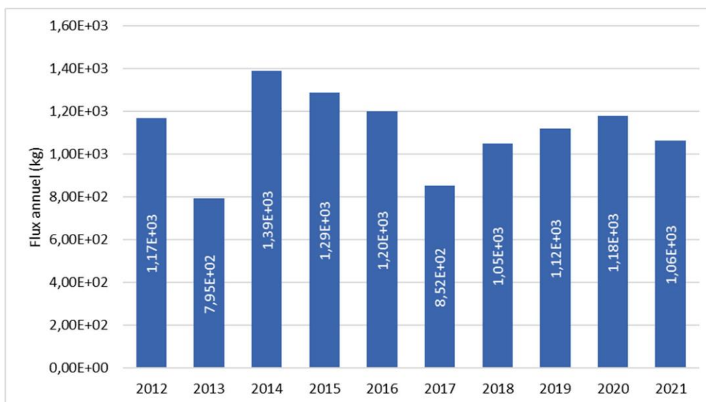
Figure 13 : Rejets annuels d'azote total sur la période 2012 – 2021 du CNPE de Saint-Laurent
