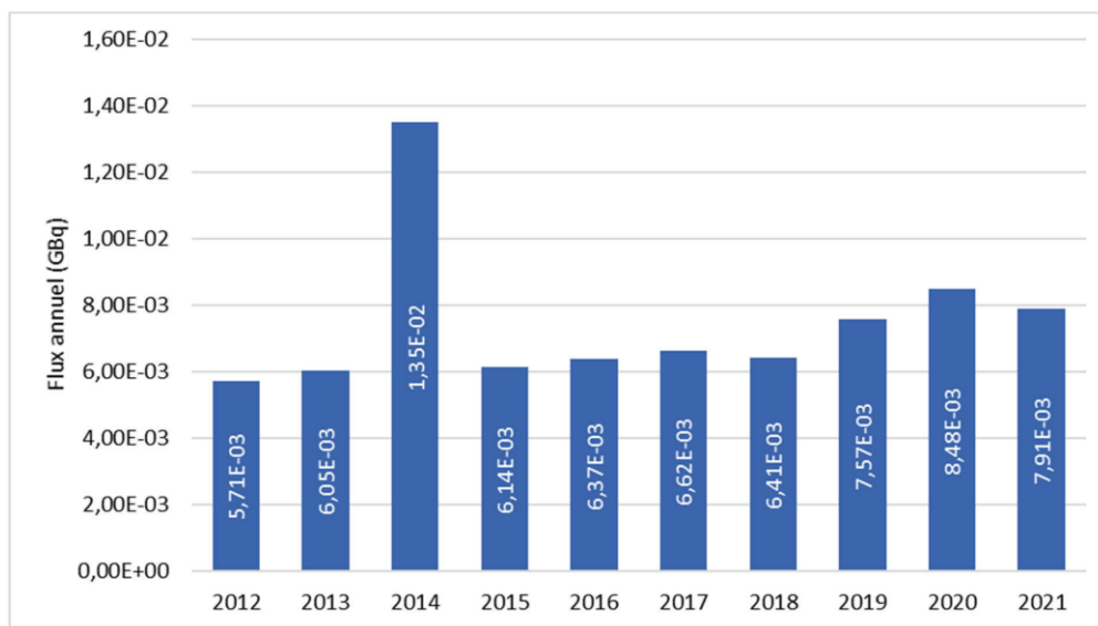
Figure 6 : Activité en iodes rejetée dans les effluents liquides du CNPE de Saint-Laurent sur la période 2012 – 2021 (GBq/an)
