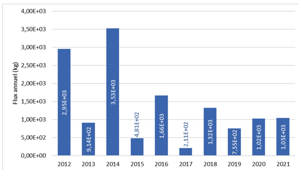
Figure 17 : Rejets annuels des nitrites issus du traitement biocide du CNPE de Saint-Laurent sur la période 2012 - 2021
