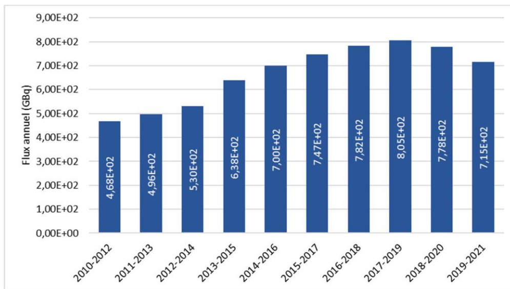
Figure 3 : Activité en tritium rejetée à l'atmosphère, moyenne sur 3 années glissantes sur la période 2012 – 2021, du CNPE de Saint-Laurent (GBq/an)
