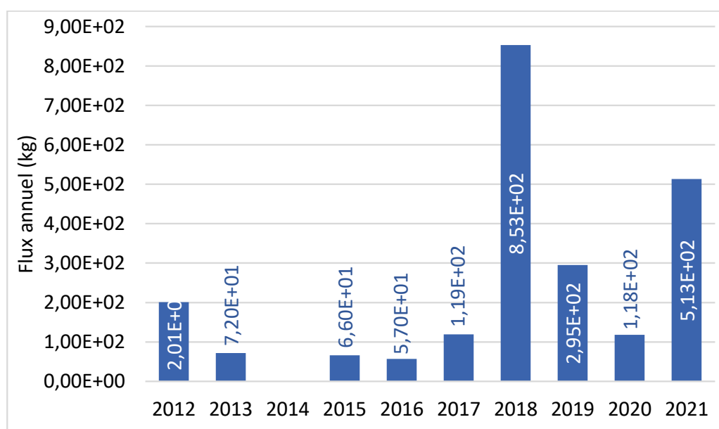
Figure 15 : Rejets annuels d'ammonium issus du traitement biocide du CNPE de Saint-Laurent sur la période 2012 - 2021
