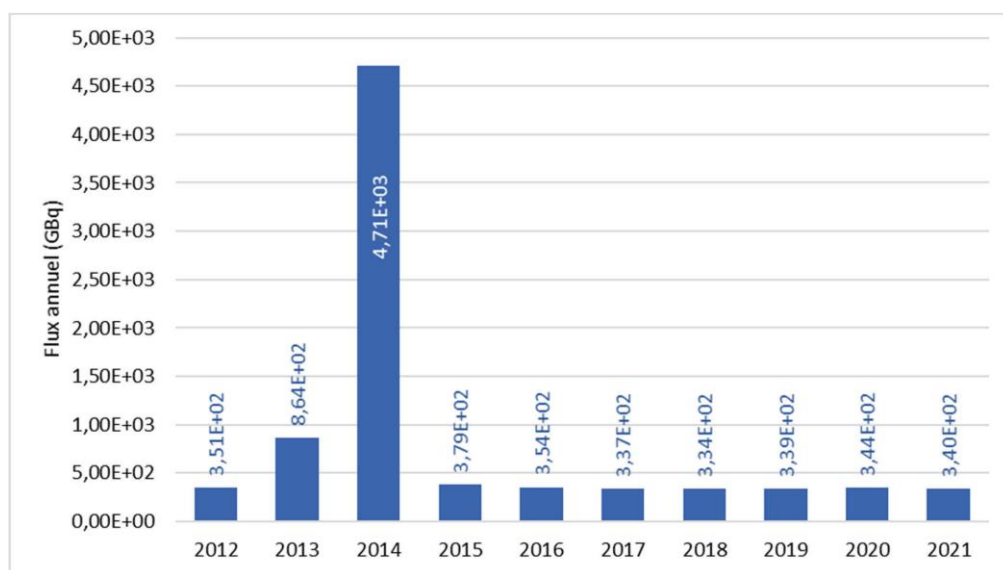
Figure 4 : Activité en gaz rares rejetée à l'atmosphère du CNPE de Saint-Laurent sur la période 2012 – 2021 (GBq/an)
