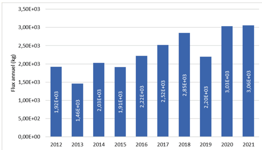
Figure 9 : Rejets annuels d'acide borique sur la période 2012 – 2021 du CNPE de Saint-Laurent
