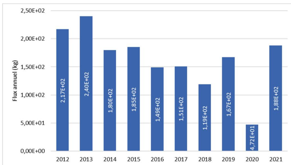
Figure 14 : Rejets annuels en phosphates du CNPE de Saint-Laurent sur la période 2012 - 2021
