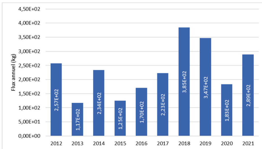
Figure 18 : Rejets annuels des AOX issus des traitements biocides du CNPE de Saint-Laurent sur la période 2012 – 2021
