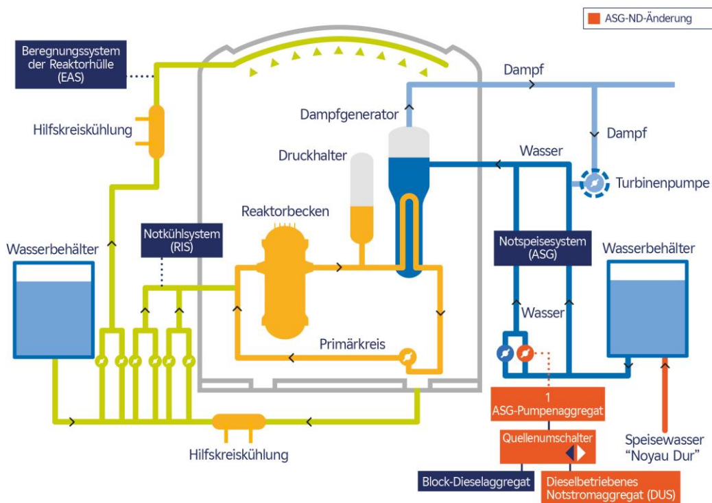
Prinzipialschaltbild der ASG-ND-Anordnung
