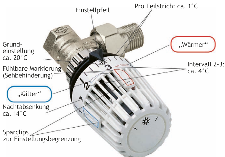
Therstatatkopf eines Thermostatventils zur Regelung der Raumtemperatur (Fa. IMI Hydronic Engineering Deutschland GmbH)
