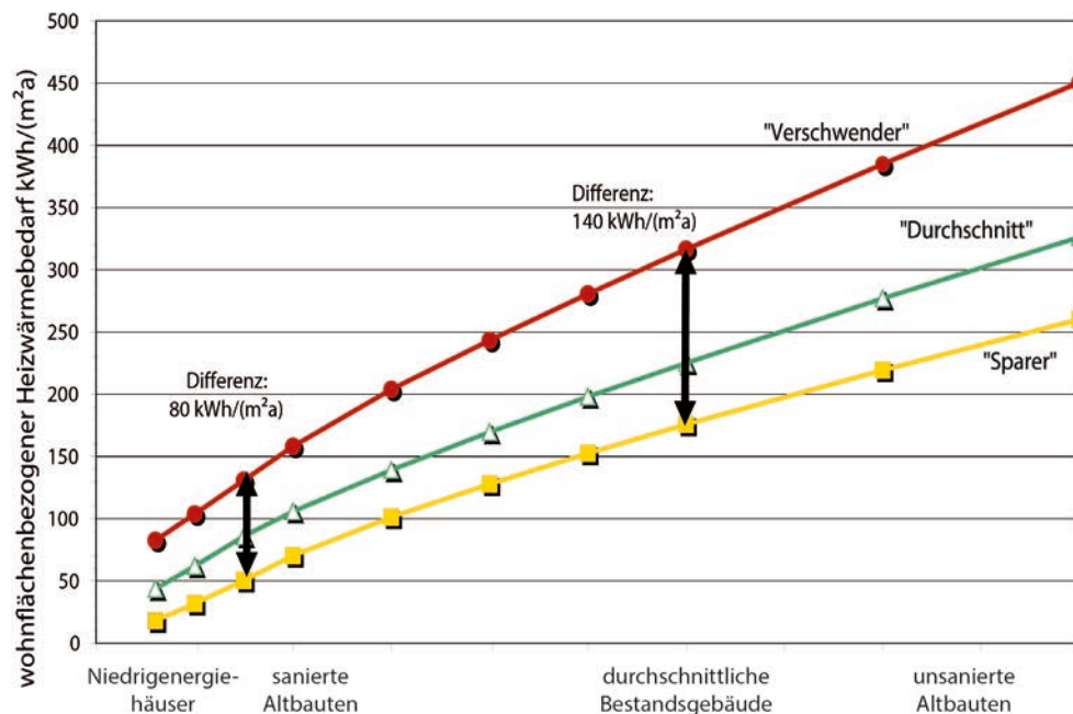
Einfluss des Nutzerverhaltens auf den Energieverbrauch (Institut Wohnen und Umwelt (IWU))
