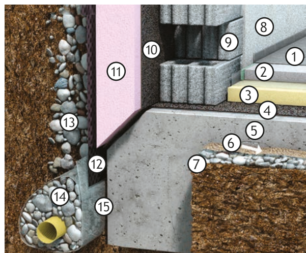
Kellersohle
