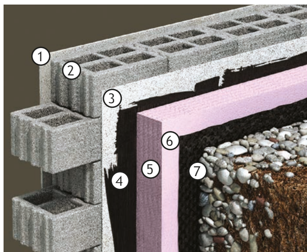
Kelleraußenwand
