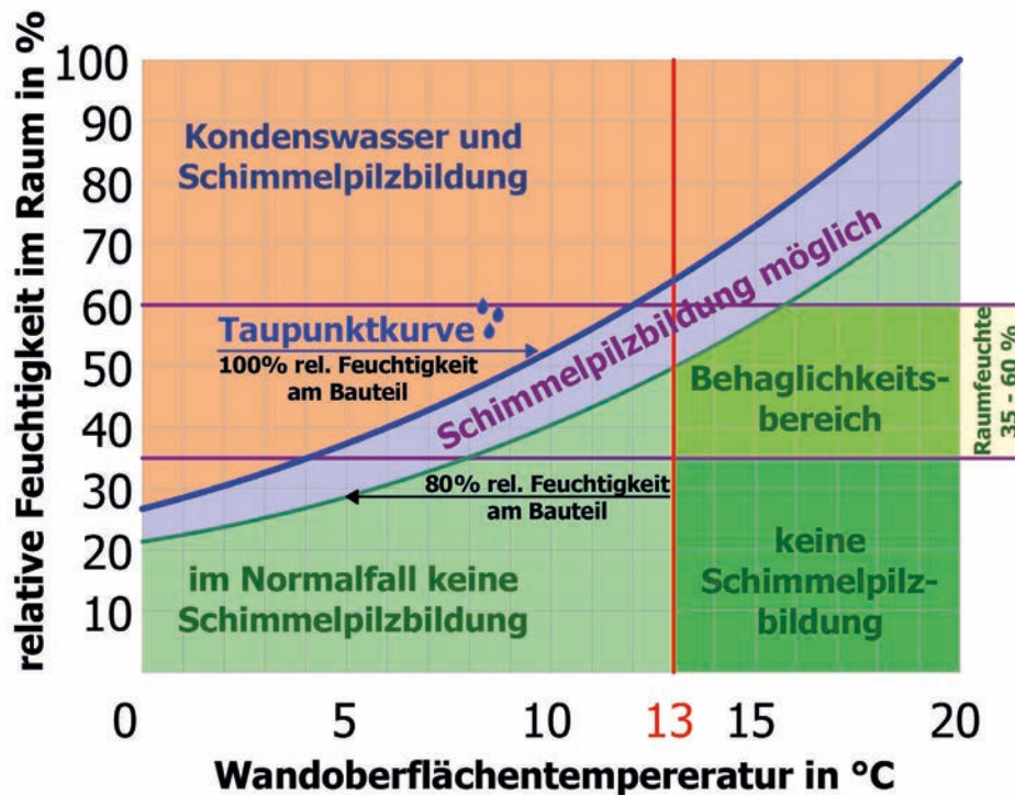
Diagramm Schimmelpilzbildung (Energieberatung Salzburg)
