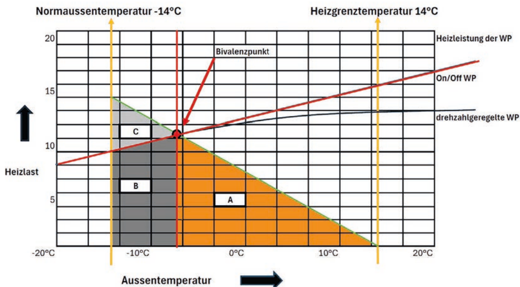
Grafische Bivalenzpunktauslegung (TERminAutor, Darstellung EBS)
